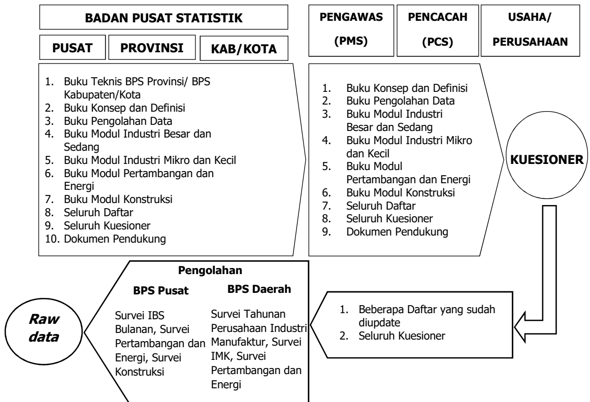
Gambar 1.1 Alur Dokumen
